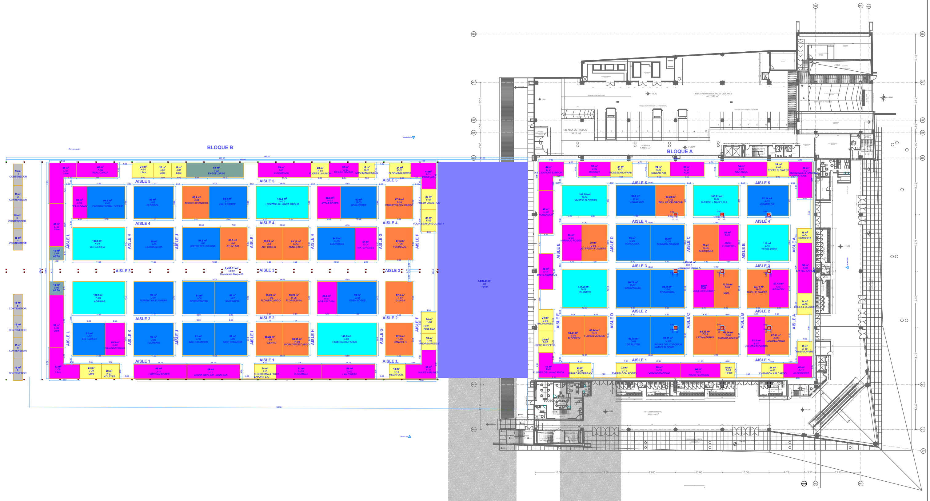
Planta Baja con Entorno
